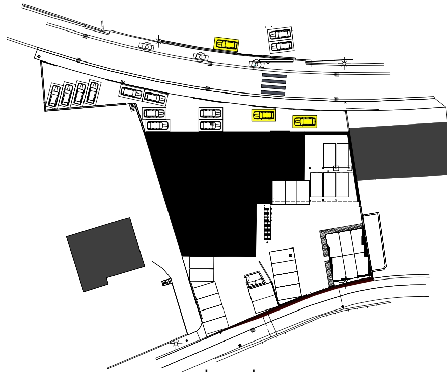
Lageplan
