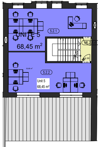
Grundriss 1.Obergeschoss
